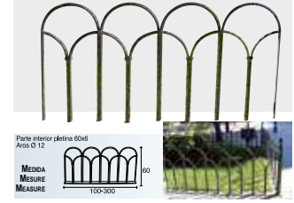
VALLA de JARDÍN Modelo 42
