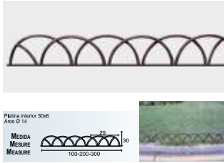
VALLA de JARDÍN Modelo 45-A Modelo 45-B
