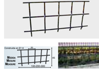
VALLA de JARDÍN Modelo 39
