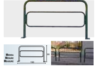
PAÑOS DE VALLA Modelo 16
