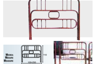
PAÑOS DE VALLA Modelo 18
